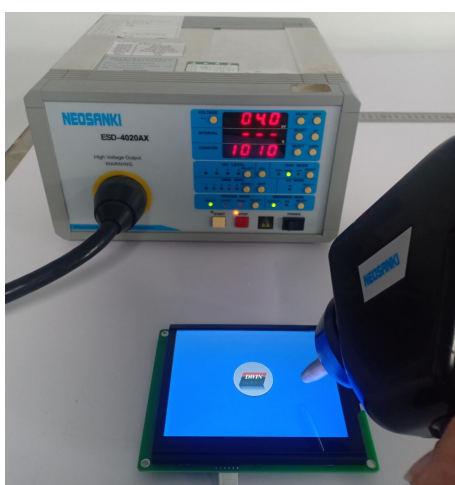
3.1 静电放电测试图
