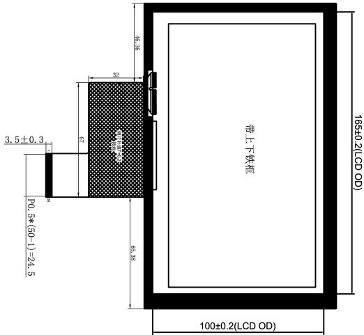
背视图
