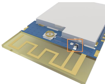
PCB antenna (default)
