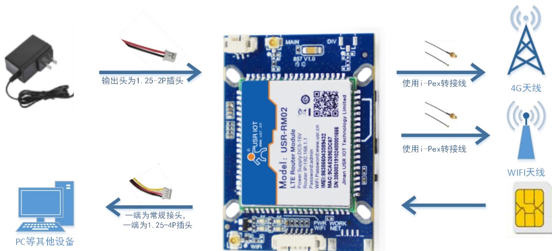
图 3 应用示意图
